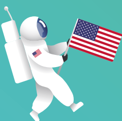
APOLLO 11 21 JUILLET 1969
